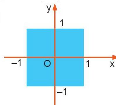
Hình 5.2. Hình vuông trong mặt phẳng tọa độ
